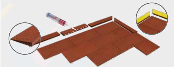
Rand- und Randeckprofile (auch mit EPDM Beschichtung)
