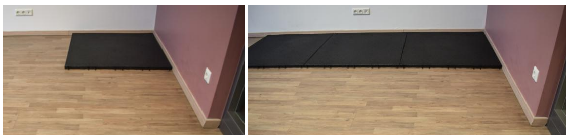
Pose des dalles le long d'un mur droit avec les connecteurs orientés vers l'avant
